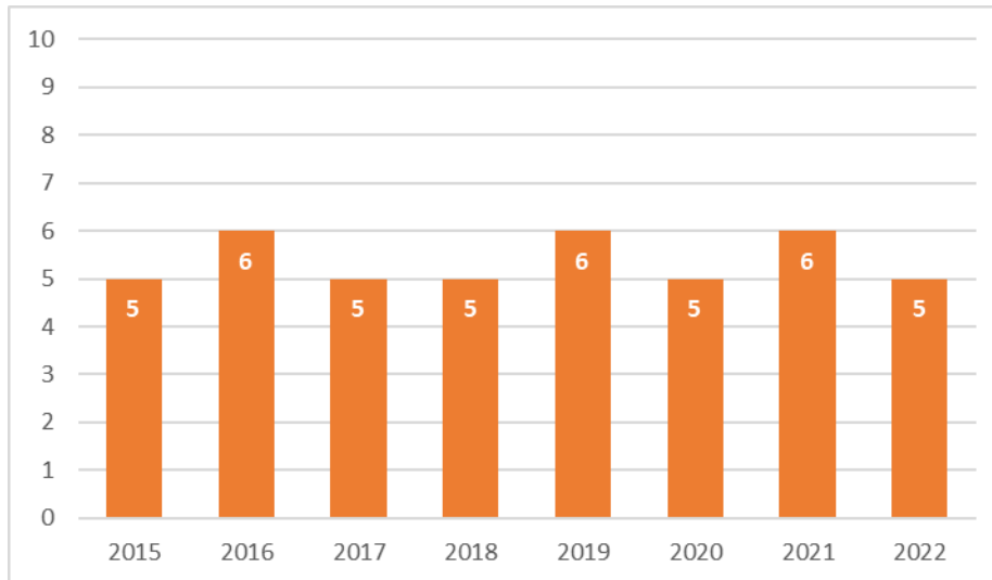
Gráfica 1: Comportamiento del IDC para el departamento de Magdalena. 2015 – 2022.
