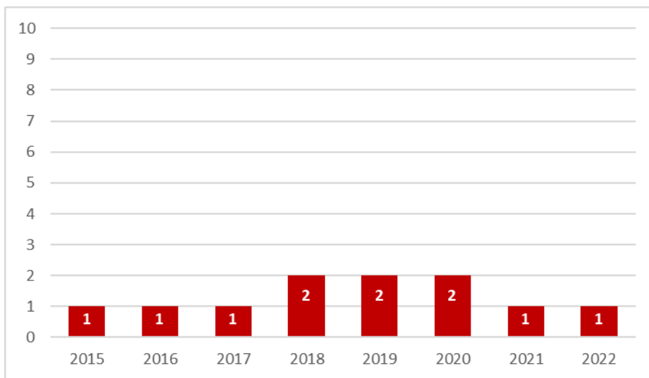
Gráfica 1: Comportamiento del IDC para el departamento de Amazonas. 2015 – 2022.
